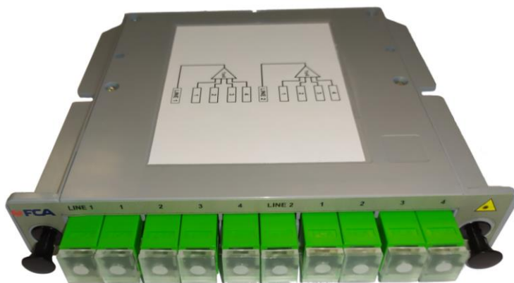
Sprzęgacz mocy 1x4 w obudowie modułowej LGX
