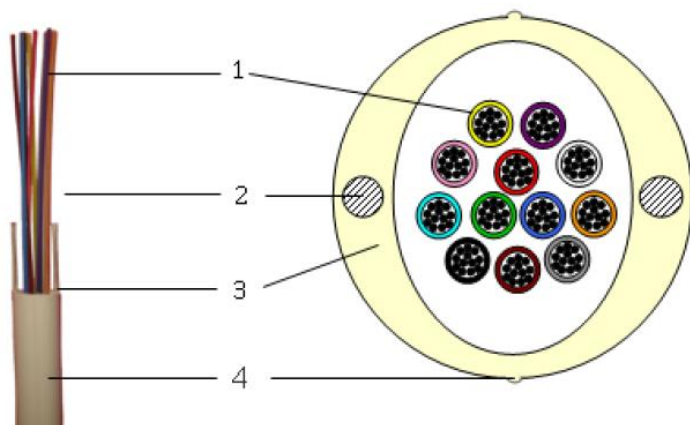
Kabel łatwego dostępu modułowy
