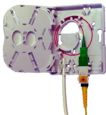
Gniazdo abonenckie serii CTB2-A
