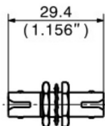
adapter A-STP-MM-HS
