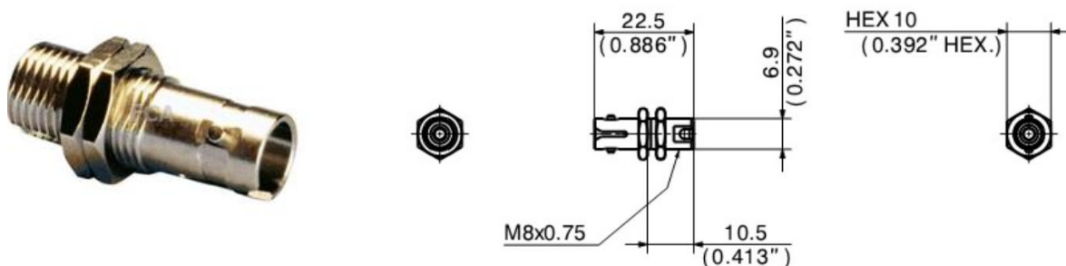
Zdjęcie oraz rysunek techniczny adaptera hybrydowego FC/ST
