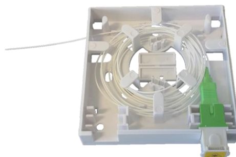
Gniazdo abonenckie serii GAP otwarte
