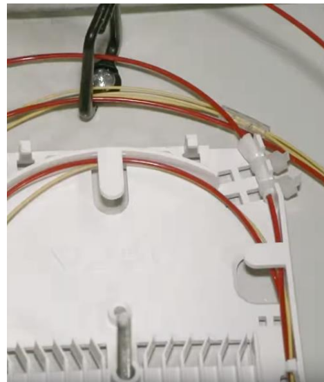
Fot.6 Mocowanie tuby światłowodowej w kasecie.
